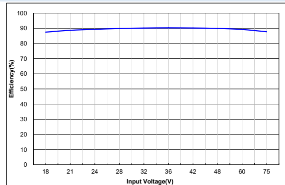
图 2: 效率值 VS 输入电压(满载)
