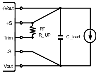
图 1. 电阻调整输出电压示意图(上调)
