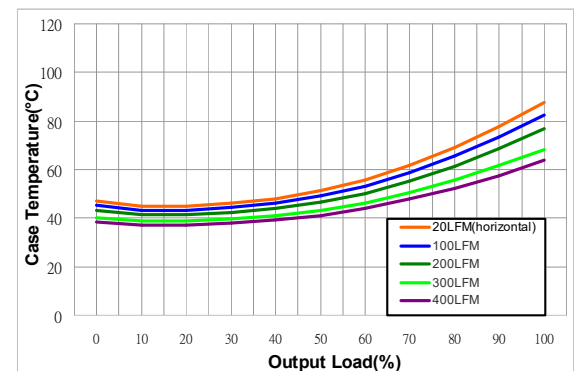
图 4: 工作亮温 VS 输出负载(满载)
